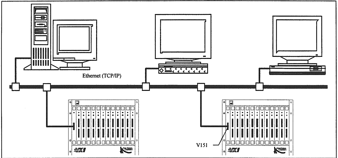
VXI mainframe
